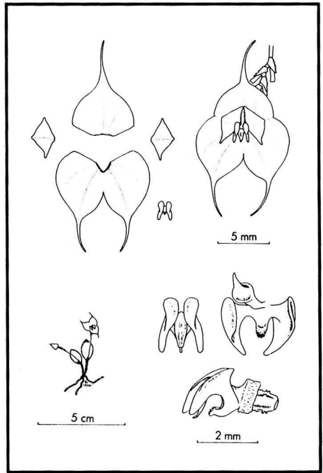
LEPANTHES TSUBOTAE
