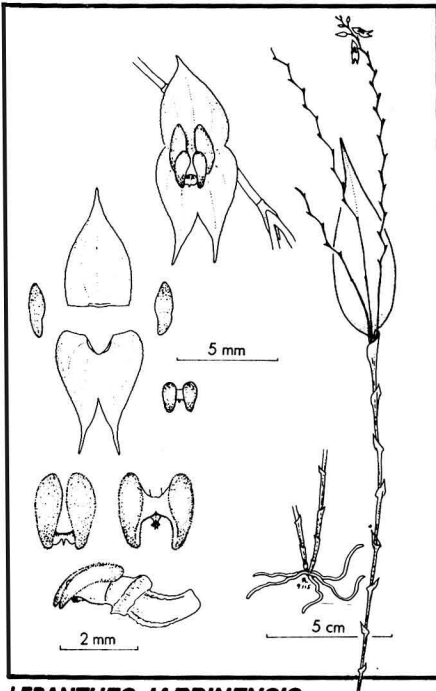
LEPANTHES JARDINENSIS
